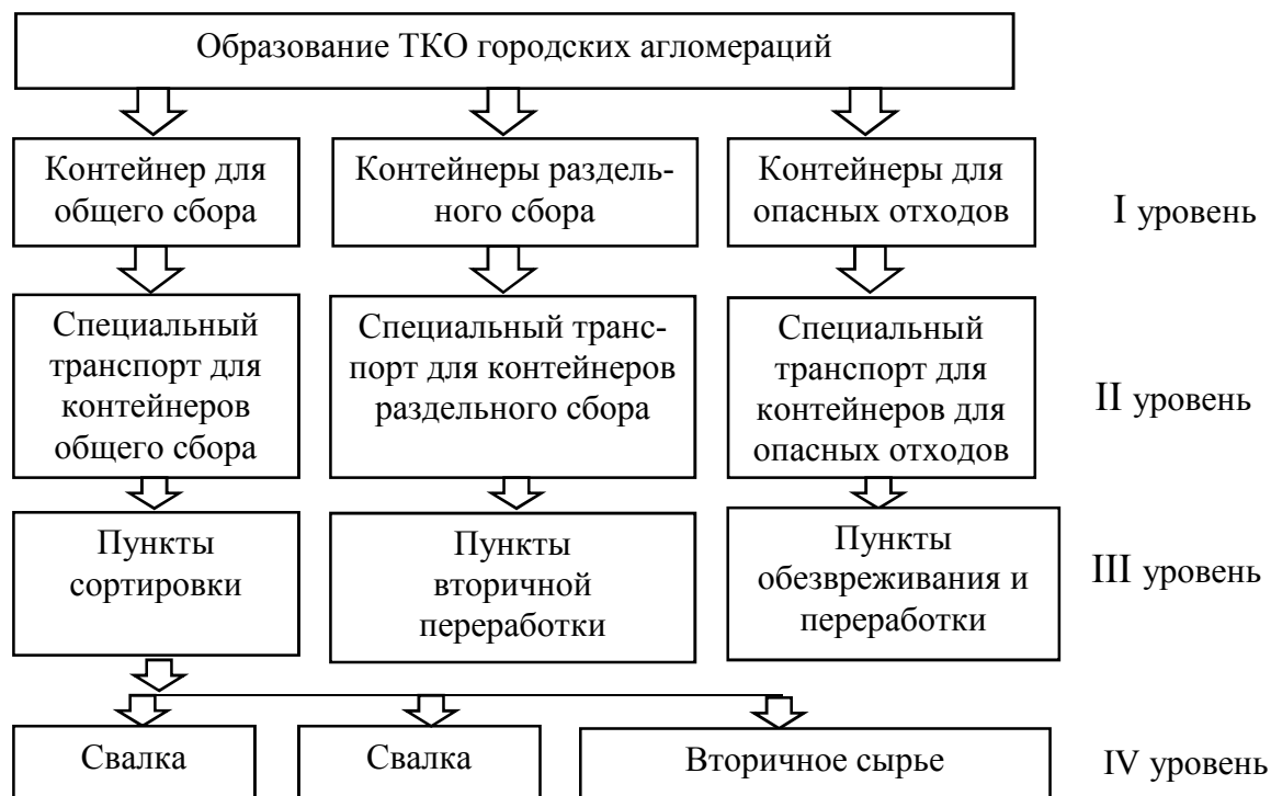
Рисунок 8 – Экологически безопасная логистическая система городских агломераций
