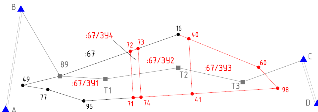
Рисунок 10. Схематический чертеж проектного разбивочного теодолитного (полигонометрического) хода.
