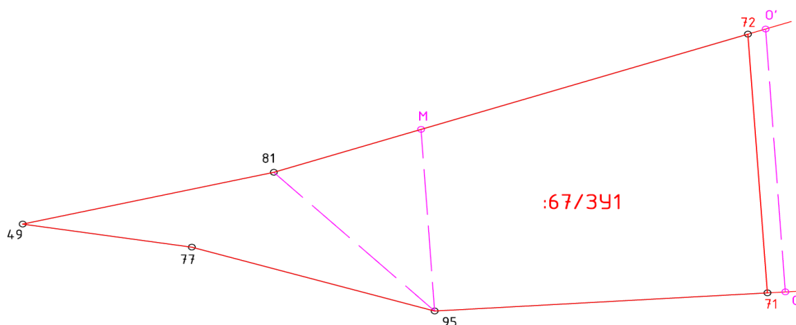
Рисунок 7. Схематический чертеж участка :67/ЗУ1
